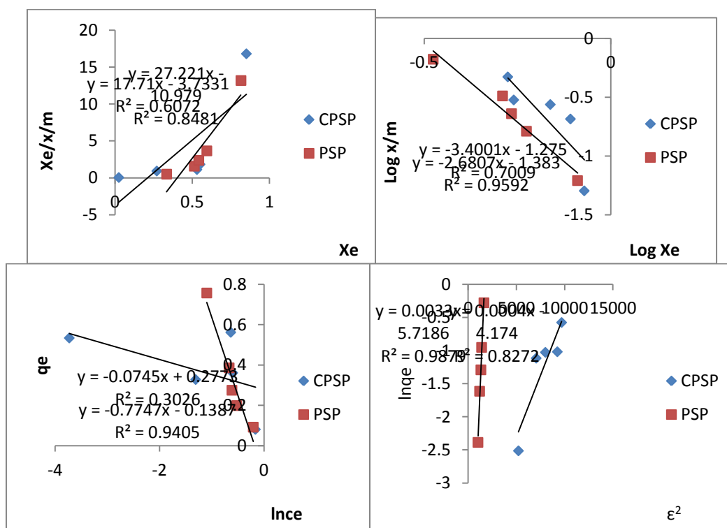
Fig. 5. Isotherm plots of (a) Langmuir, (b) Freundlich, (c) Temkin and (d) D-R
